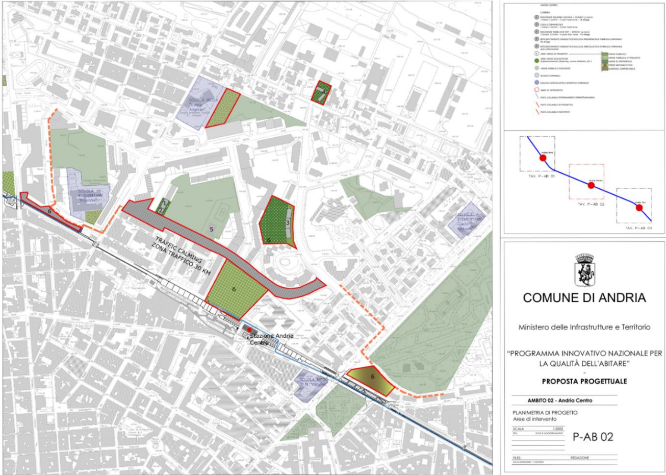
Figura 2.2 – Progetto stazione Andria centro
